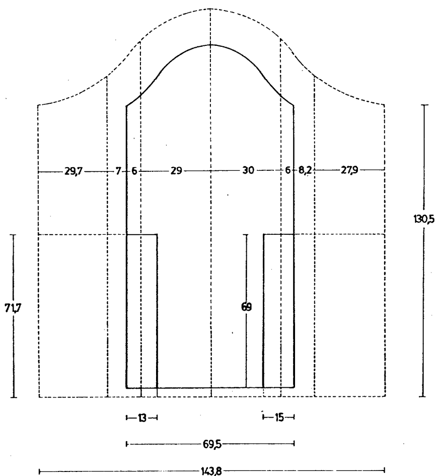
Fig. 4.—Triptico Flamenco de Agaete. Panel central. Reconstrucción. Medidas. Elaboración propia.
