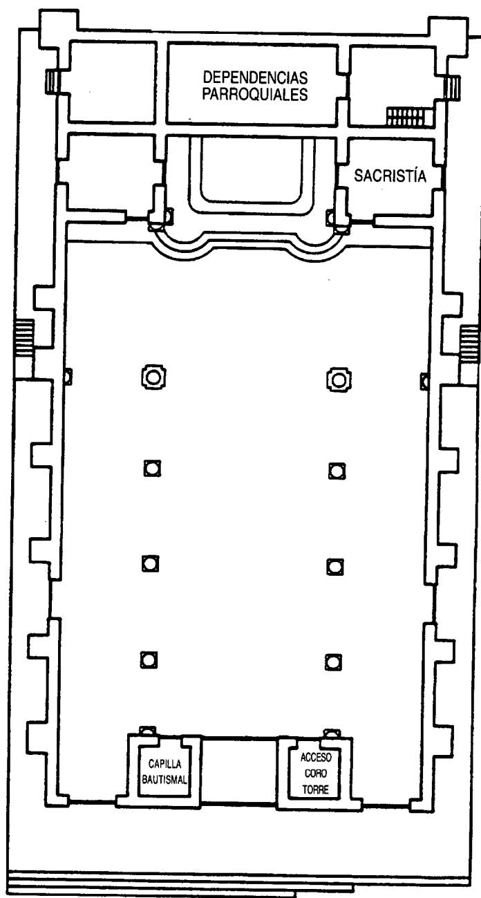
FIGURA 4.—Iglesia matriz de Nuestra Señora de la Concepción. Estado actual. Plano de don Francisco de la Torre y Sarmiento. Elaboración propia.
