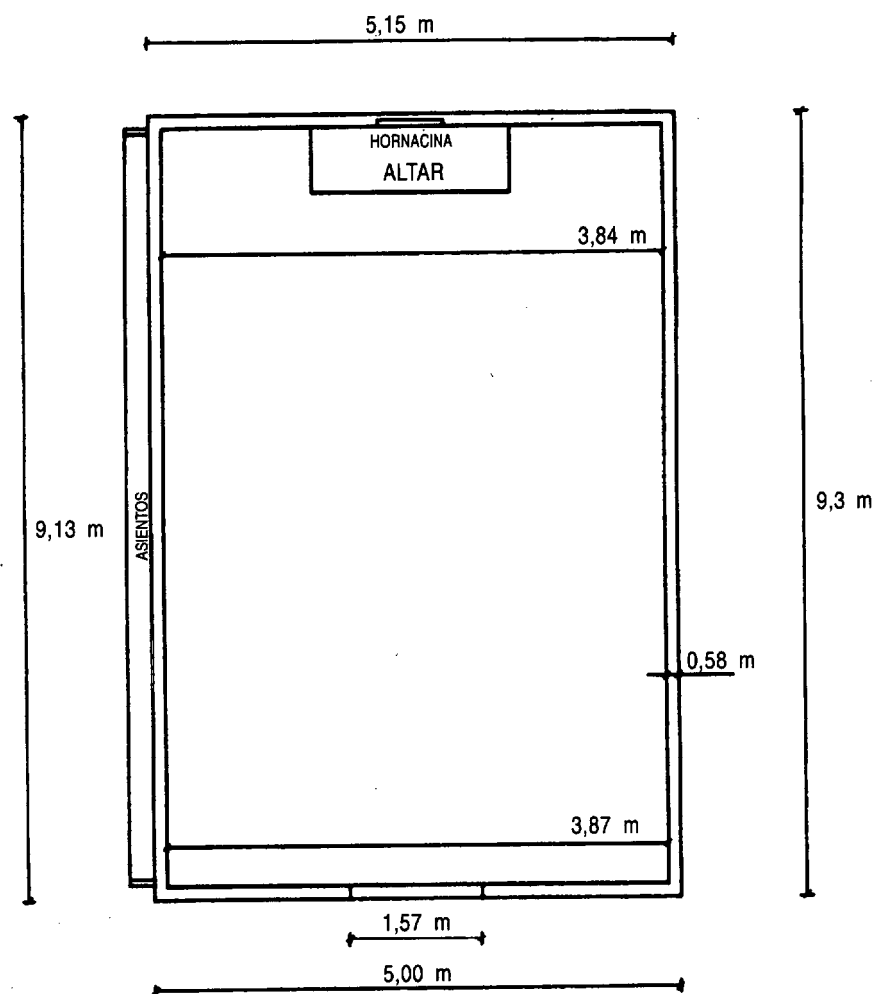
FIGURA 6.—Ermita de San Sebastián. Estado actual. Primera mitad del siglo XVII. Plano del autor.
